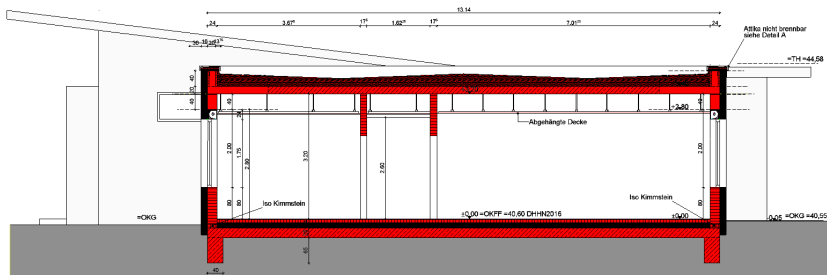
SCHNITT A-A'
